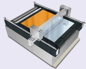
パネルレベルスリットコーター Slit coater for panel level packages LC-M550G
